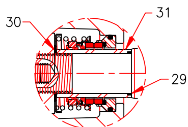
ÍTEM 2 SELLO MECÁNICO
