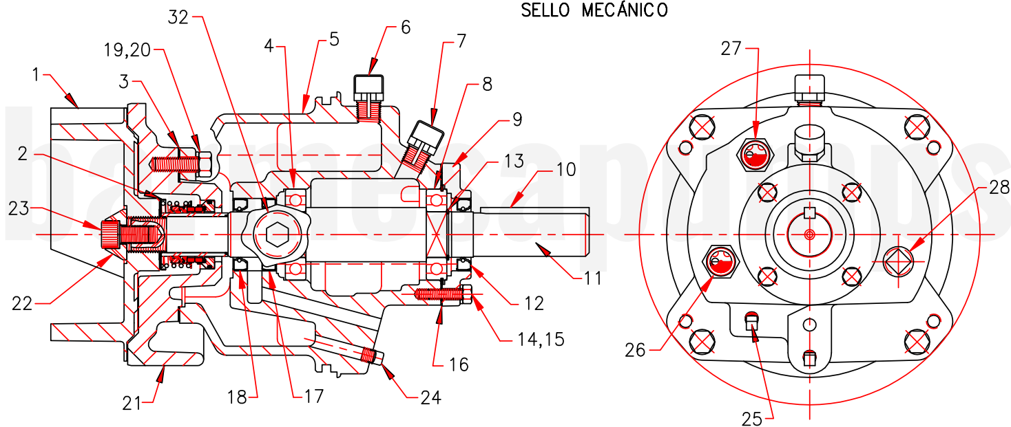
DIBUJO SECCIONAL DE EXTREMO MOTRIZ SH3-U
