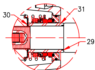
ÍTEM 2 SELLO MECÁNICO
