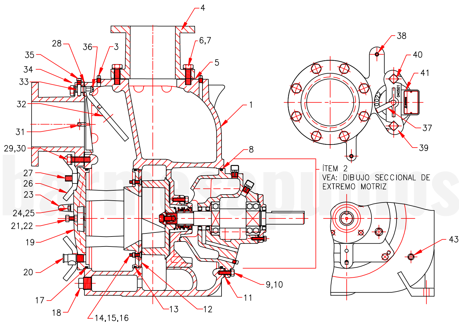
BOMBA SH6-U, DIBUJO SECCIONAL
