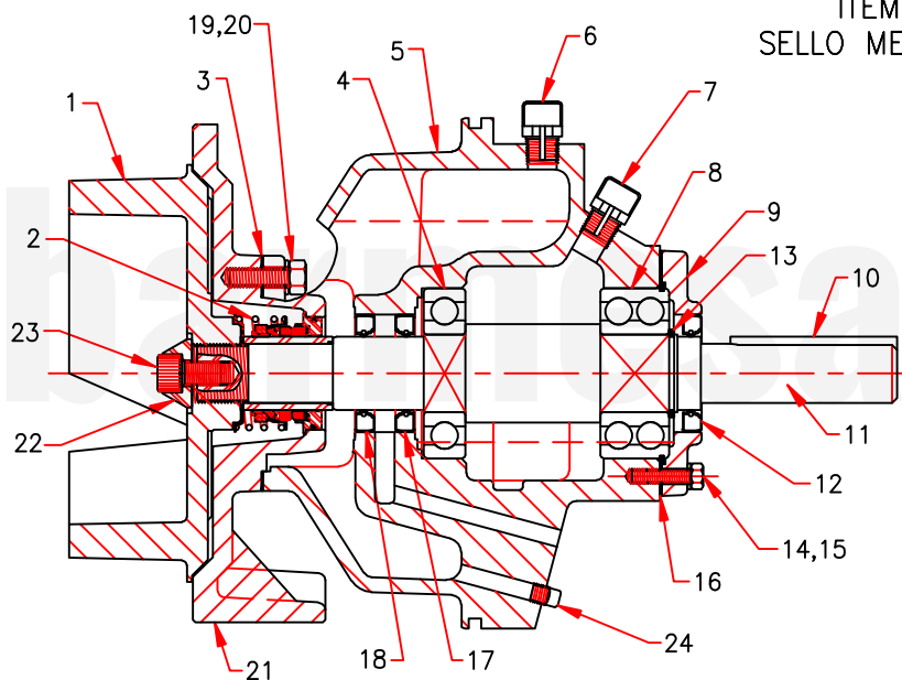
DIBUJO SECCIONAL DE EXTREMO MOTRIZ SH6-U
