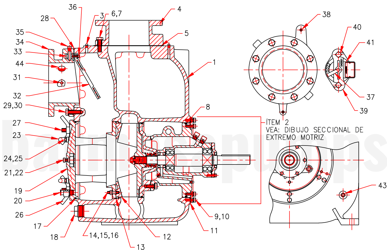
BOMBA SH8-U, DIBUJO SECCIONAL
