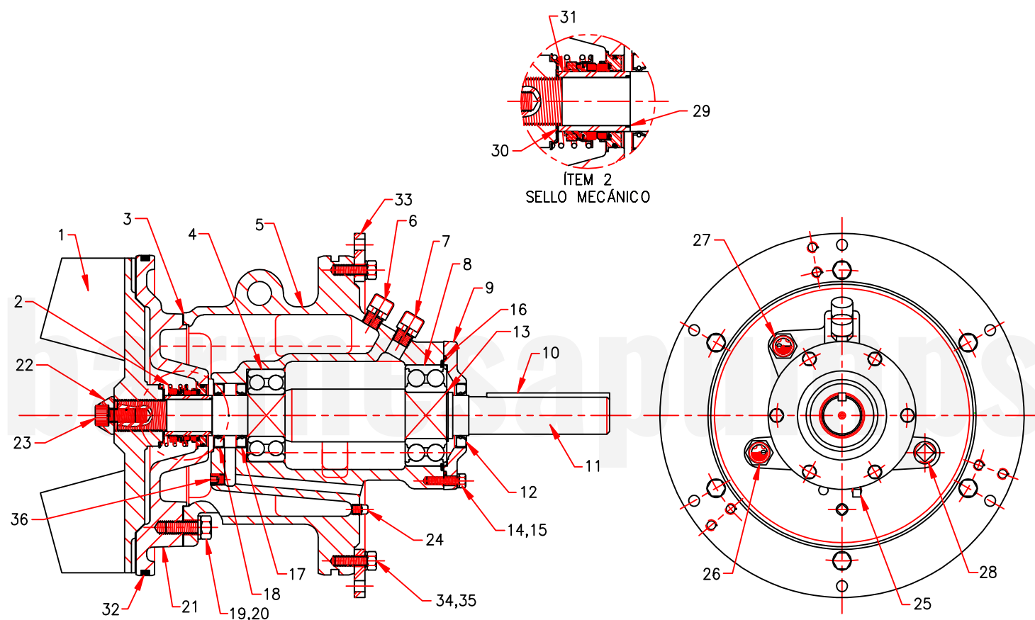
DIBUJO SECCIONAL DE EXTREMO MOTRIZ SH8-U
