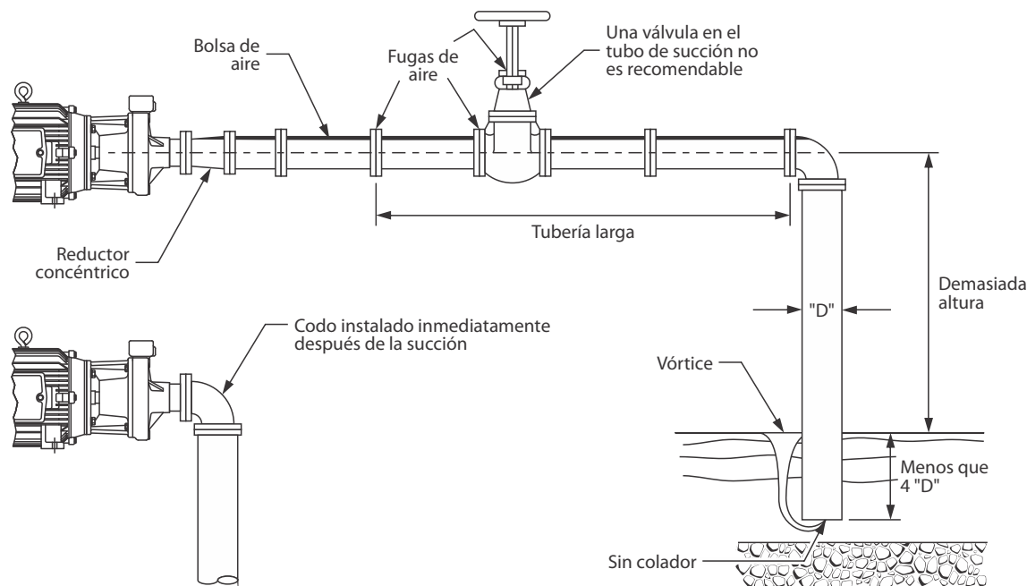
Figura 2 Instalación incorrecta.
