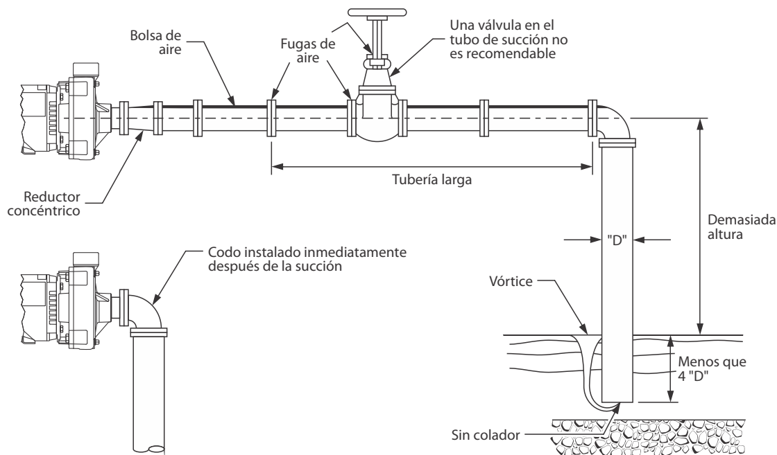
Figura 2 Instalación incorrecta.
