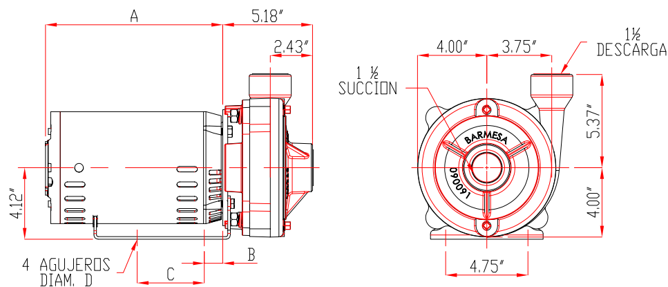
DIMENSIONAL MODELO IC 1½ CON BASE
