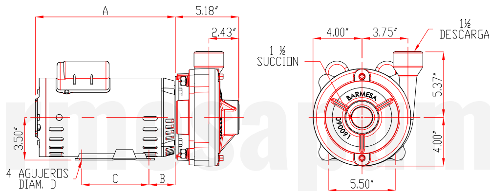
DIMENSIONAL MODELO IC 1½ CON BASE
